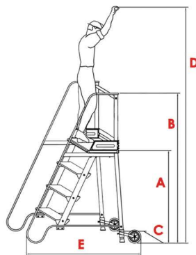
Peldaño ancho de 150 mm con sistema de fijación anti-torsión al largo
